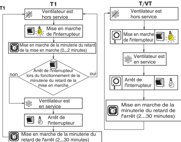
SILENCE 100 T/T1, SILENCE 125 T/T1, SILENCE 100 VT, SILENCE 125 VT
