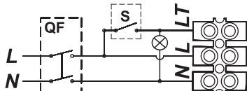
SILENCE 100 VT, SILENCE 125 VT
